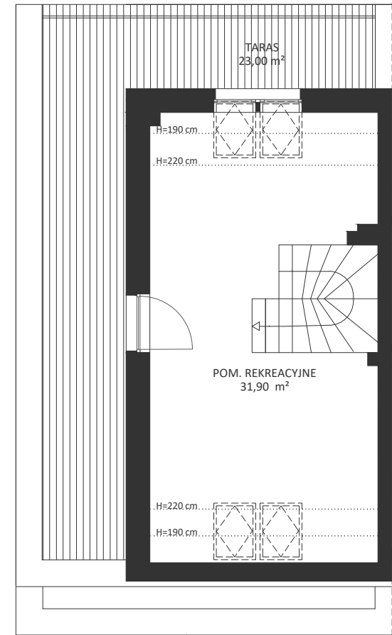
PODDASZE
